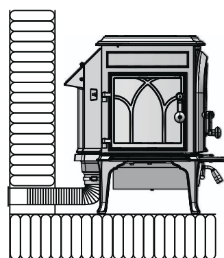
Fig. 9a Par un mur
