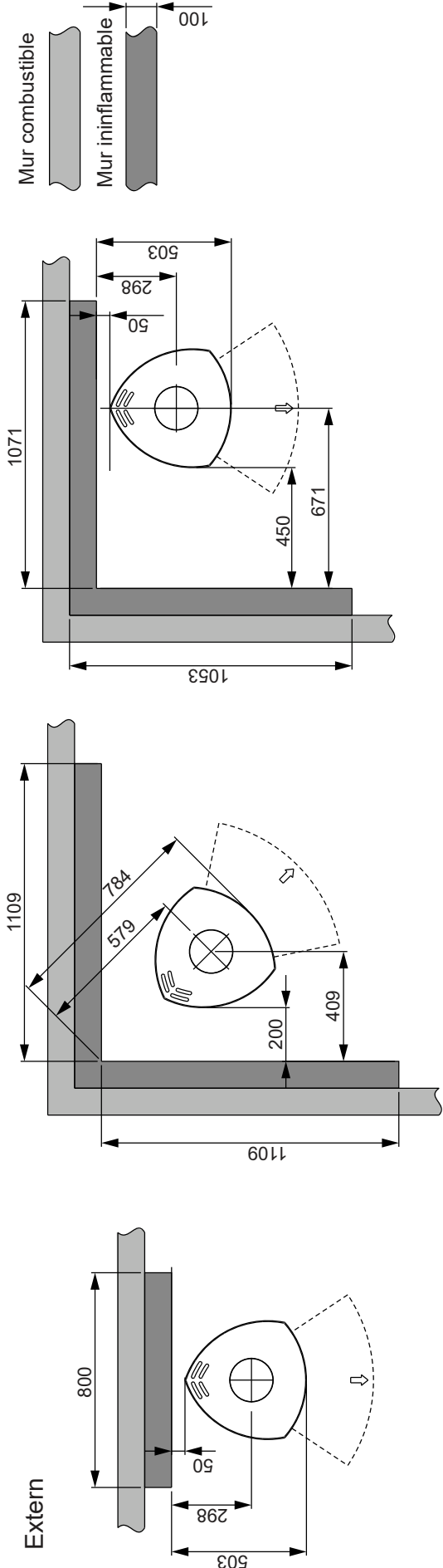
Jøtul F 370 Advance - Distance minimale par rapport au mur en matériau combustible protégé par un pare-feu
