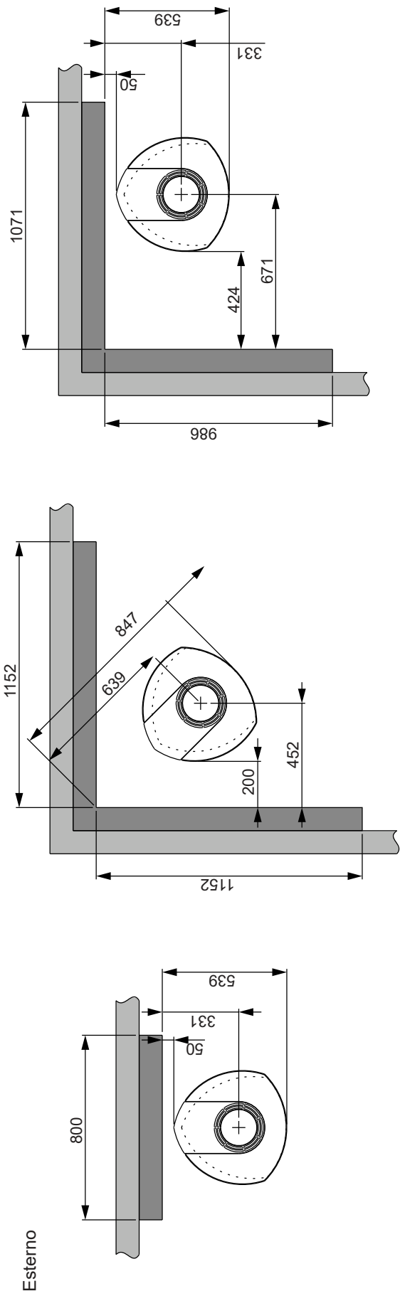
Jøtul F 377 Advance - Distancia mínima a una pared de material no combustible
